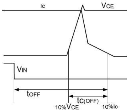
(b) 关断
