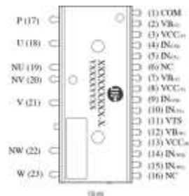
PIN1-PIN23
