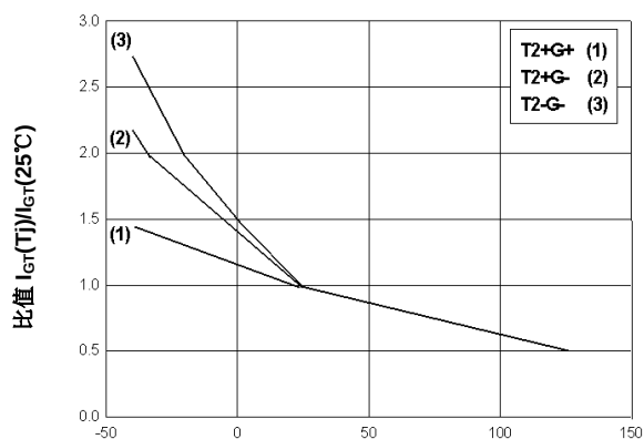
结温 T_j(^{\circ}C)
