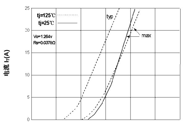
通态压降 V_{TM}(V)
